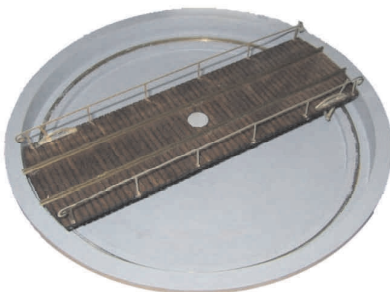
878005 12,8m drejeskive/Drehscheibe/turntable elektrisk drev, Electroantrieb/eletric drive For AC and DC Sporlængde/ Länge der Bühne/length og tracks: 150 mm
