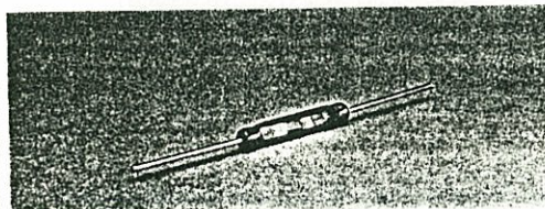
1700 SRK-Wechselkontakt Gesamtlänge 44 mm, Länge des Glaskörpers 16 mm. Außen \varnothing 2,5 mm, Belastbarkeit 0,8 Amp. bei 50 000 Schaltspielen
