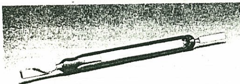
1500 SRK-Wechselkontakt Gesamtlänge 70 mm, Länge des Glaskörpers 54 mm. Außen \varnothing 1,5 mm, Belastbarkeit 2 Amp. bei 50 000 Schaltspielen
