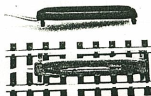
1823 Schalkontakt für N-Gleise ohne Schotterbett 34 × 8 × 4,5 mm
