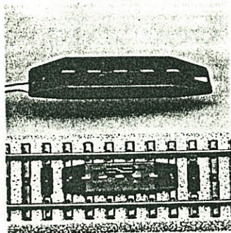
1820 Schalkontakt für H0-Metallgleise mit Punktkontakten 42 × 13 × 7 mm
