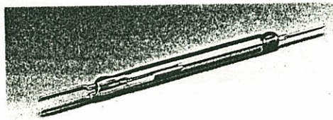
1600 SRK-Umschaltkontakt Maße wie für 1500, Belastbarkeit 1 Amp. bei 50 000 Schaltspielen
