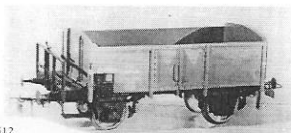
FFJ PU 1313 med bremseplatform, byggesæt.
