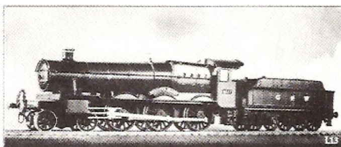
1213 GWR eksprestogslok. type "Grange".
