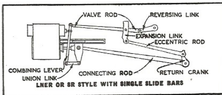
3064 Heusingerstyring. (uden cylindre) ætset nysølv med krydshoved og nitter. sæt til to sider.
