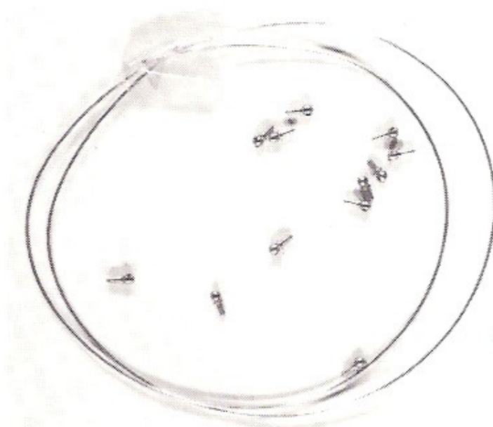
3023 Lokomotivgelænder. Består af: 12 holdere i messing og 30 cm. nysølv tråd.
