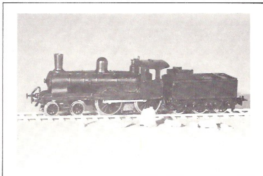
1001 DSB damplokomotiv litra C i hvidmetalbyggesæt komplet med motor (2 skinne jævnstrøm) og transfer.
