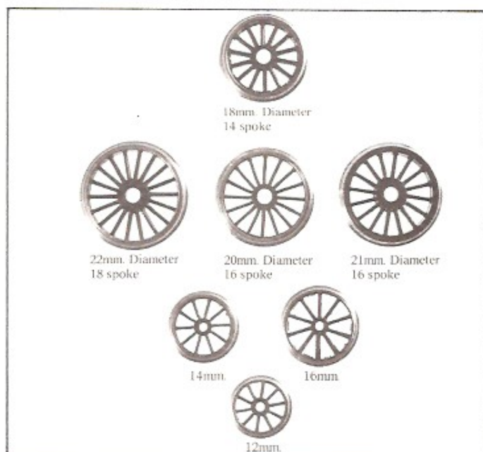
3002 Tenderhjulpar/løbehjulpar med aksel.
