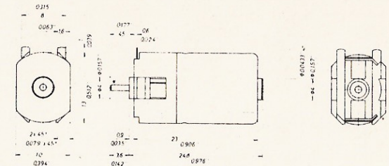
3015 Bühler motor 3-polet, 12 volt jævnstrøm.
