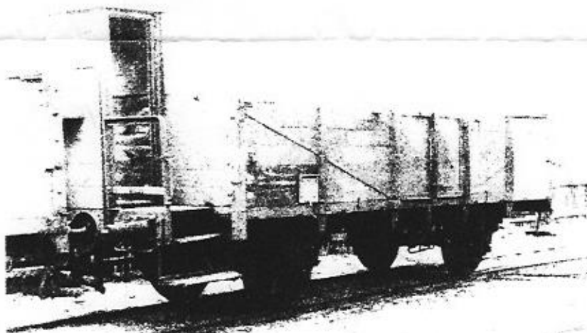
Åben godsvogn m/ bremsehus KRB Pj 95 i tyskerbrun farve. Vognen blev udrangeret i 1963.
